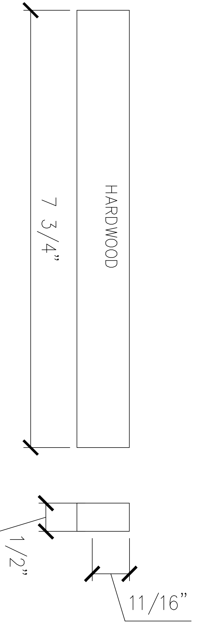
SECTION F1 SCALE FULL
