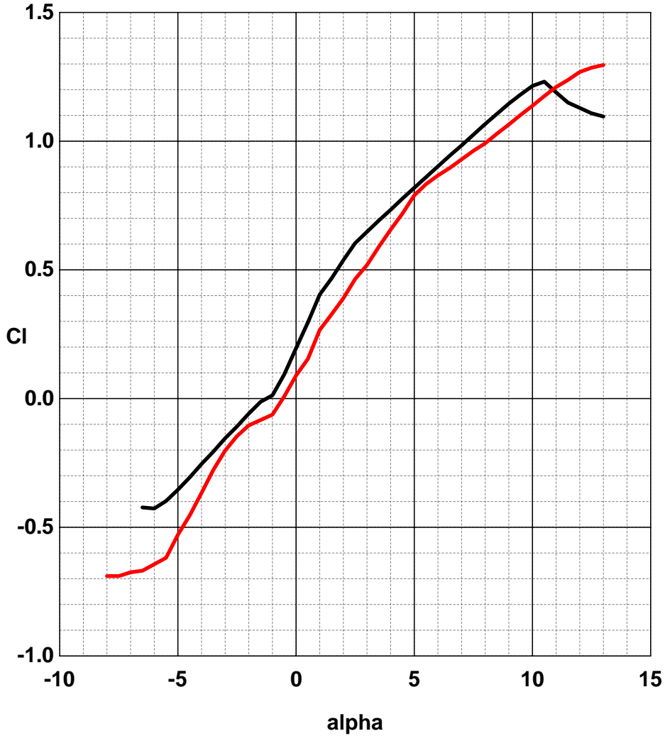
Cl(alpha):
