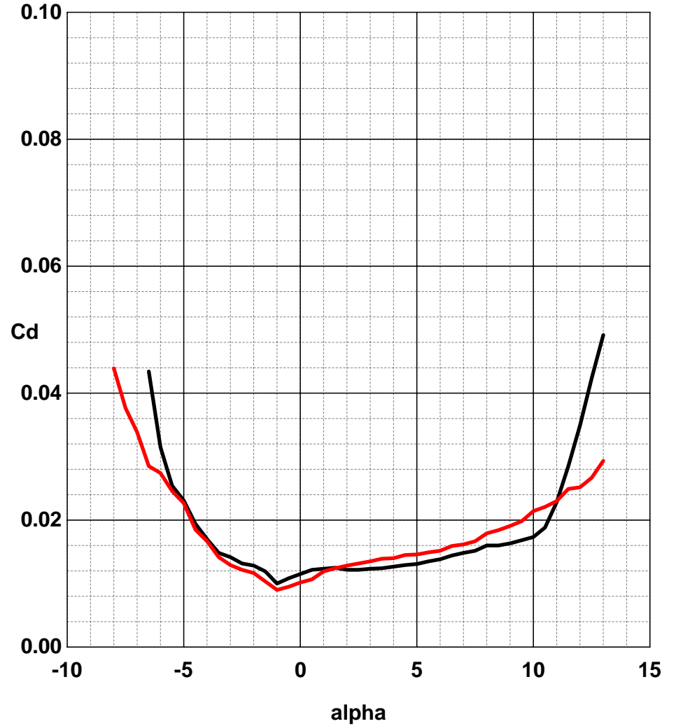
Cd(alpha):
