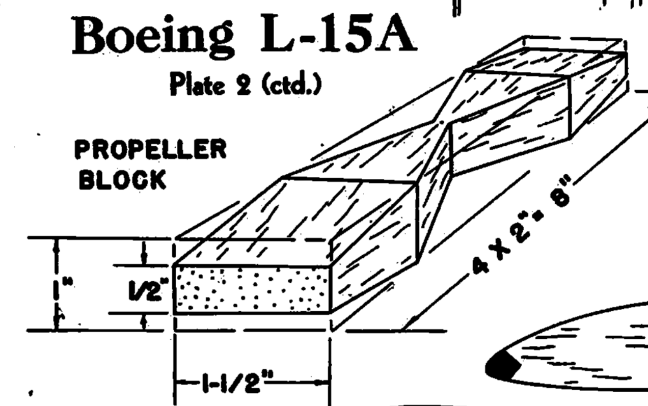
Boeing L-15A Plate 2
